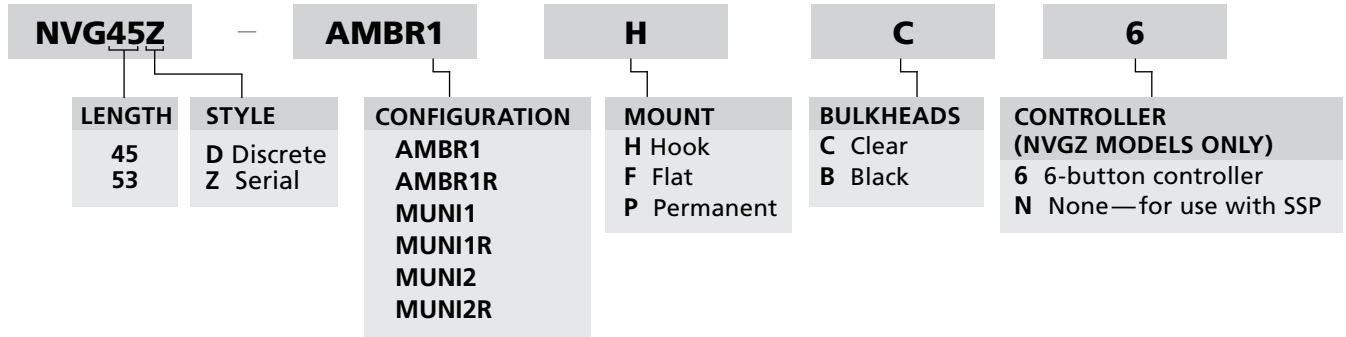
AMBR1 All Amber, SignalMaster
