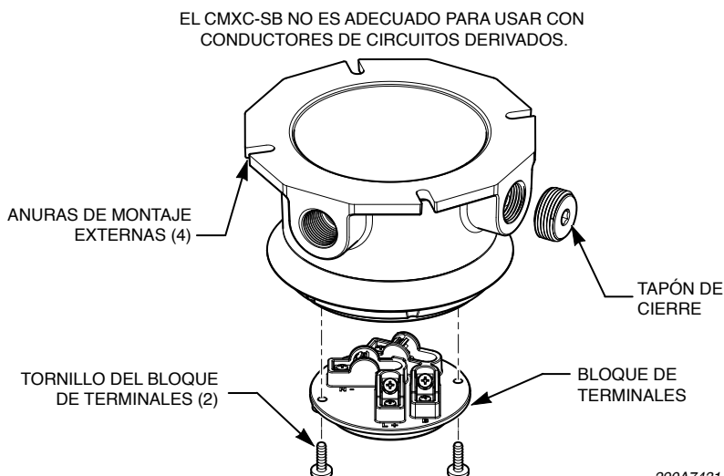
Figura 2 Vista expandida del montaje para techo
