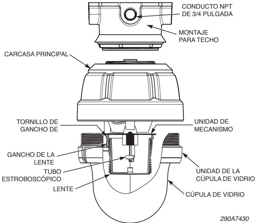
Figura 1 Vista expandida de la luz
