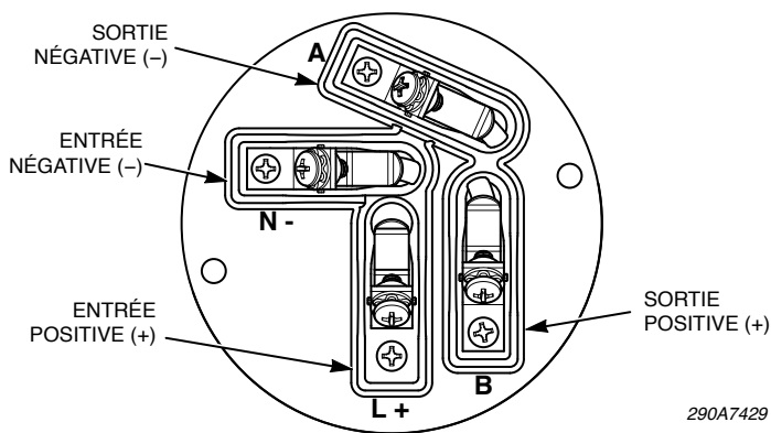
Figure 3 Bloc de jonction
